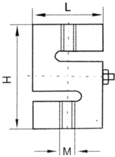
S-образный датчик
